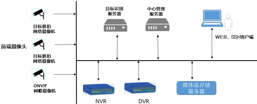
图 3-1 典型的目标识别系统架构图
